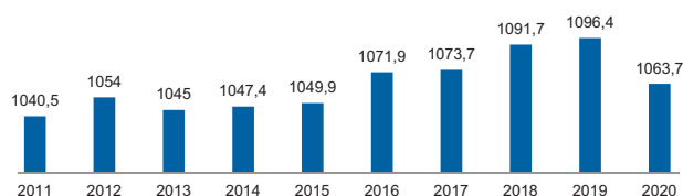
Рисунок 10.18 — Динамика выработки электроэнергии, 2011–2020 гг., млрд кВт·ч
