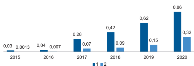
Рисунок 10.19 — Динамика доли ветровых и солнечных электростанций в структуре установленной мощности (1) и в выработке электрической энергии в ЕЭС Российской Федерации (2), %
